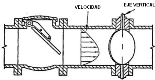
FIGURA 4. VALVULA DE RETENCION AGUAS ARRIBA
