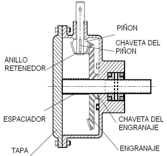
FIGURA 10. ENGRANAJE PIÑON (Abre-Derecha)
