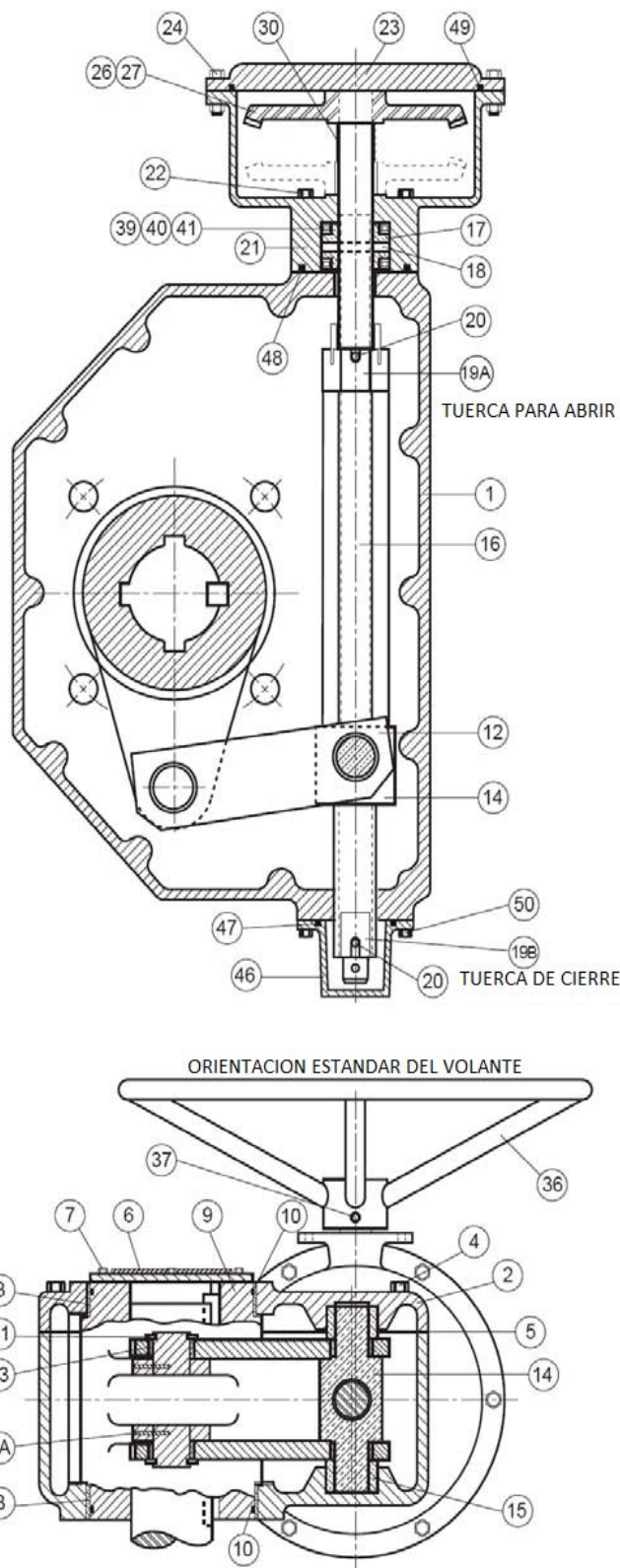
FIGURA 9. CONSTRUCCION DEL ACTUADOR DESLIZANTE
