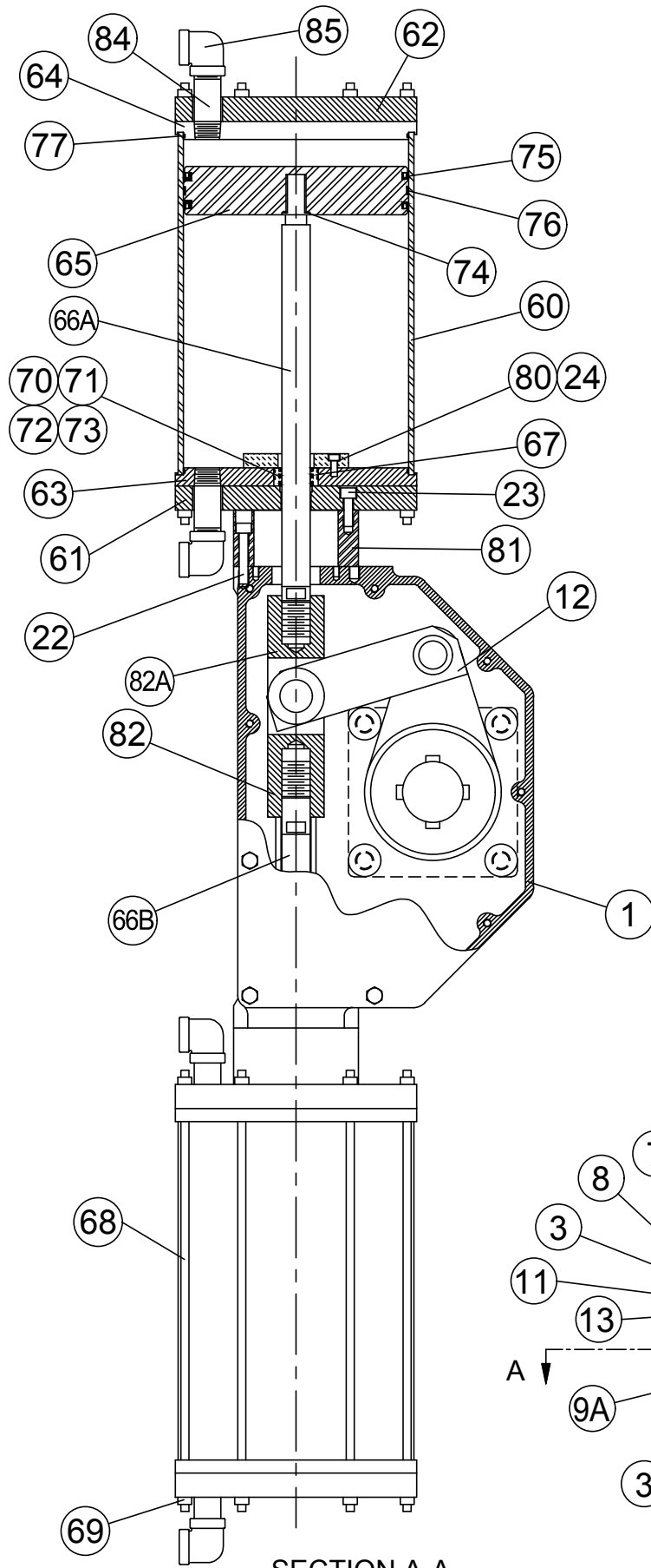
SECTION A-A
